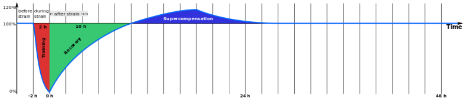
Schaubild: Superkompensationsprinzip 1
